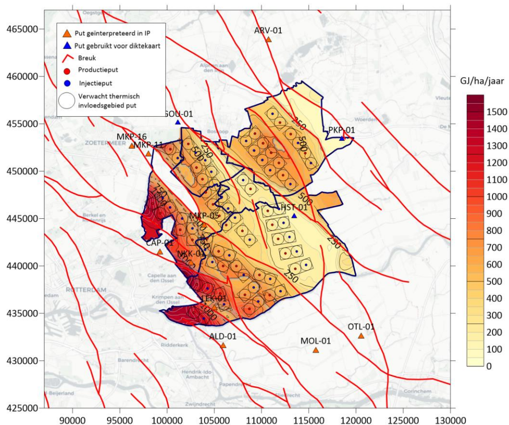
Figuur 3.8 | Inpassing van 38 geothermische doubletten in de regio Midden-Holland voor het bepalen van de "Potential Recoverable Heat".
