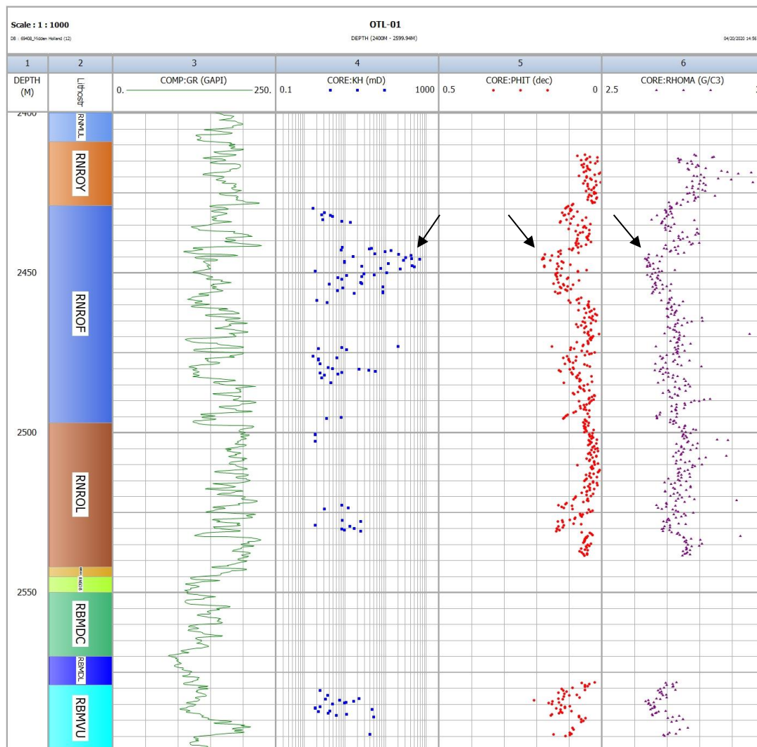
Figuur 4.3 | Kerndata OTL-01 put. Zie tussen 2442-2450 mAH een zone in het Röt Randzandsteen Laagpakket met verhoogde permeabiliteit, deze correspondeert met verhoogde porositeit ( >0.1 ) en een lagere dichtheid <2.6 g/cm 3 (zwarte pijlen). Kolom 1 geeft de diepte weer langs het boortraject. Kolom 2 geeft de lithostratigrafie weer: RNROY = Boven-Röt Randkleisteen Laagpakket, RNROF = Röt Randzandsteen laagpakket, RNROL = Onder-Röt Randkleisteen Laagpakket, RNSOC = Solling Kleisteen Laagpakket, RNSOB = Basale Solling Zandsteen Laagpakket, RBMDL = Detfurth Kleisteen Laagpakket, RBMDL = Onder-Detfurth Zandsteen Laagpakket, RBMVU = Boven-Volpriehausen Zandsteen Laagpakket. Kolom 3 geeft de gamma ray weer, een deflectie naar links is representatief voor zandsteenlaag en een deflectie naar rechts is representatief voor kleisteenlaag. Kolom 4 zijn kernmetingen van de permeabiliteit, kolom 5 zijn kernmetingen van de porositeit en kolom 6 zijn kernmetingen van de dichtheid.
